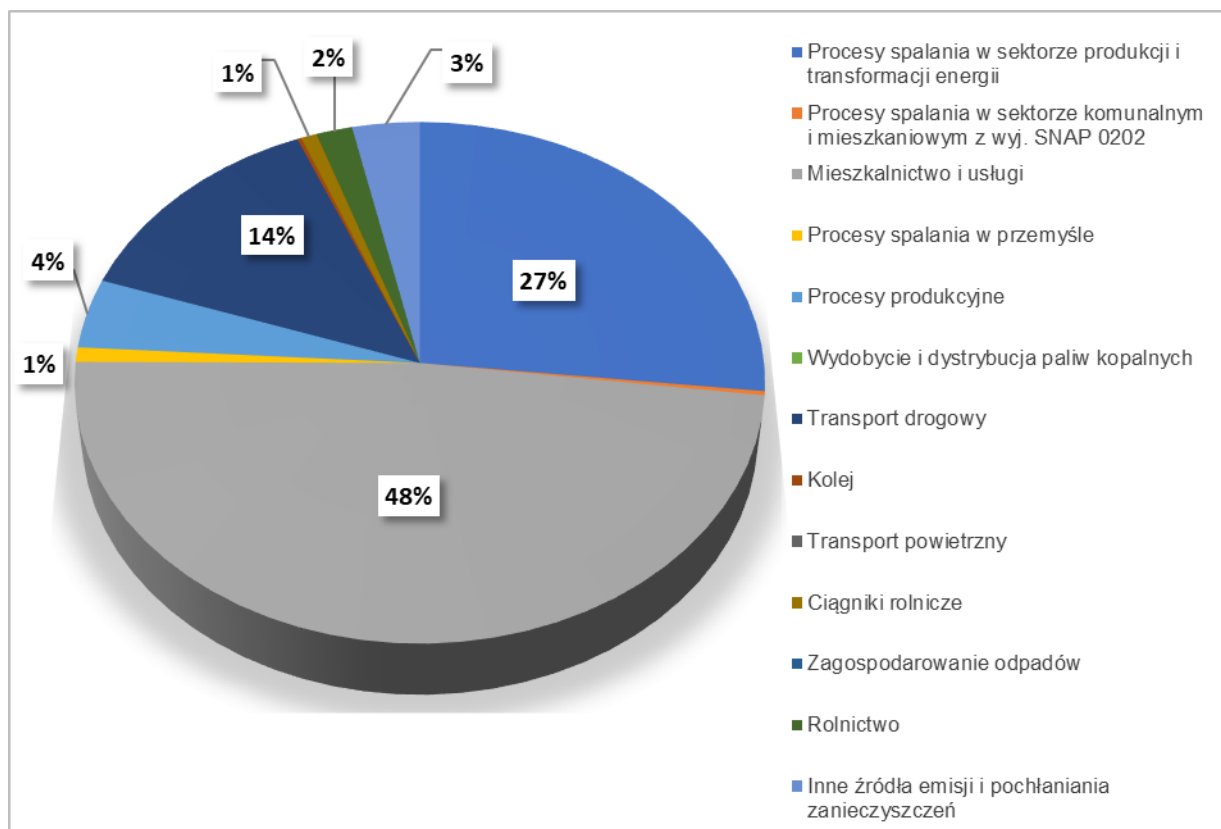
Rysunek 1-23 Udziały [%] poszczególnych rodzajów emisji, wg. kategorii SNAP w łącznej emisji pyłu zawieszonego PM10 w strefie miasta Elbląg w 2018 r.
