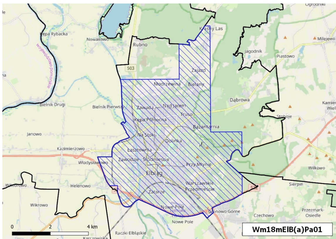
Rysunek 1-20 Obszar przekroczeń średniorocznego poziomu docelowego B(a)P w strefie miasto Elbląg w 2018 r. (kod obszaru Wm18mELB(a)Pa01)
