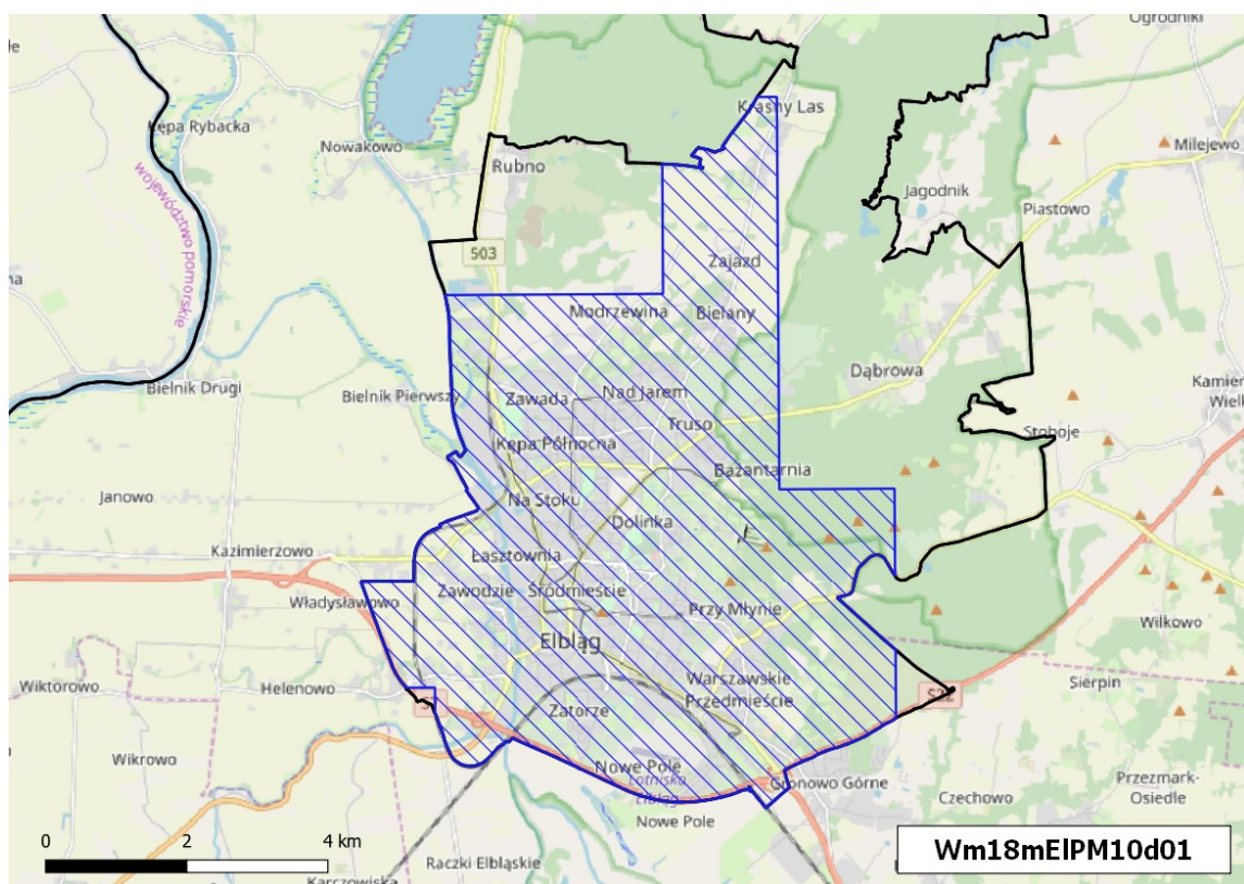
Rysunek 1-19 Obszar przekroczeń średniodobowego poziomu dopuszczalnego pyłu zawieszonego PM10 w strefie miasto Elbląg w 2018 r. (kod obszaru Wm18mELPM10d01)
