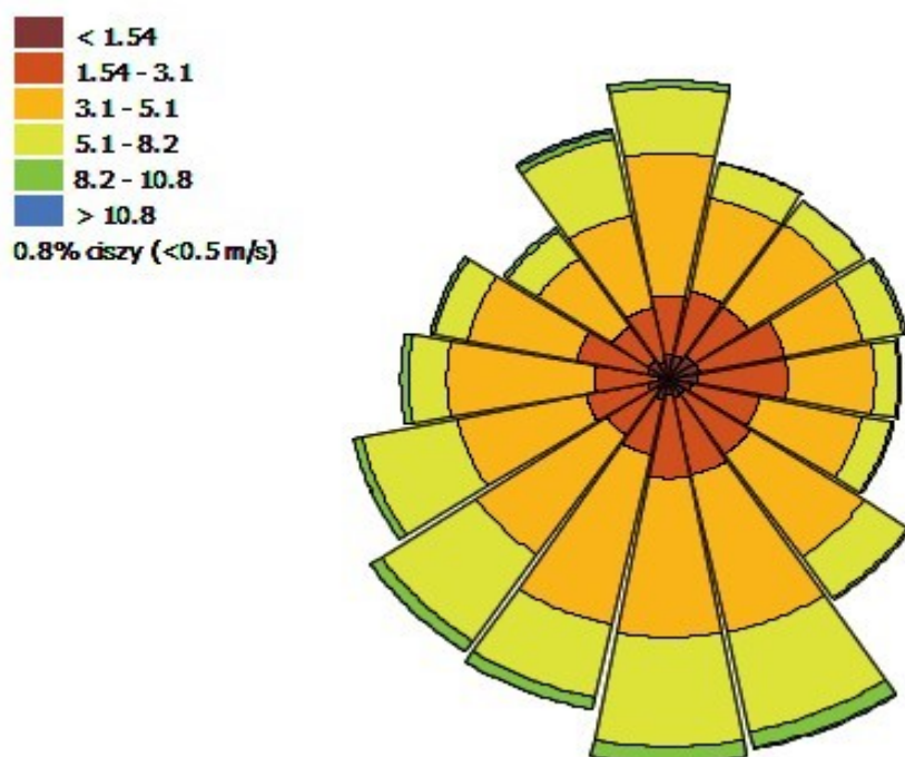
Rysunek 1-11 Rozkład kierunków i prędkości wiatru dla strefy miasto Elbląg w 2018 r.
