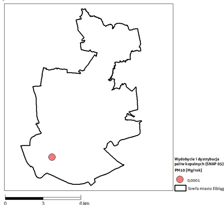
Rysunek 1-30 Rozmieszczenie oraz ładunki emisji punktowej pyłu zawieszonego PM 10 w procesie wydobywania i dystrybucji paliw kopalnych (SNAP 05) w strefie miasto Elbląg w 2018 r.
