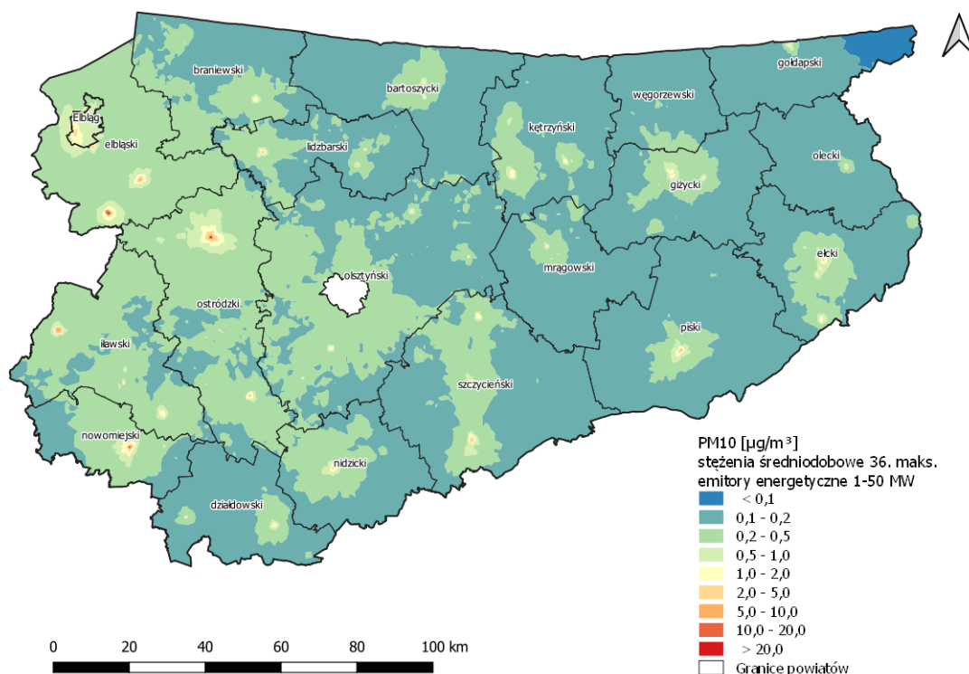
Rysunek 1-43 Średniodobowe stężenia pyłu zawieszonego PM10 (36 max) ze źródeł o mocy 1-50 MW w województwie warmińsko-mazurskim w 2018 r.
