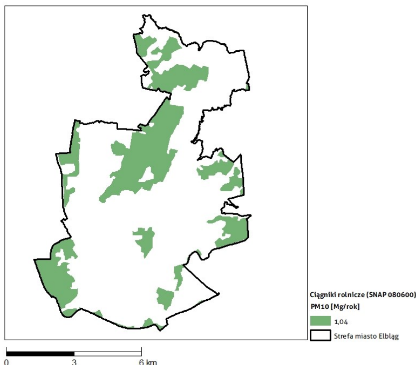
Rysunek 1-33 Rozmieszczenie oraz ładunki emisji powierzchniowej pyłu zawieszonego PM10 wyemitowane przez ciągniki rolnicze (SNAP 080600) w strefie miasto Elbląg w 2018 r.
