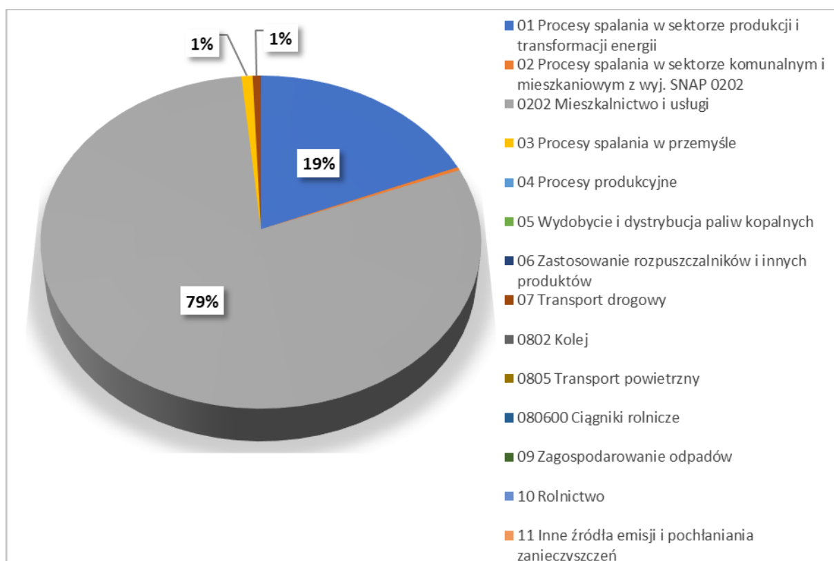
Rysunek 1-24 Udziały [%] poszczególnych rodzajów emisji, wg. kategorii SNAP w łącznej emisji B(a)P w strefie miasta Elbląg w 2018 r.
