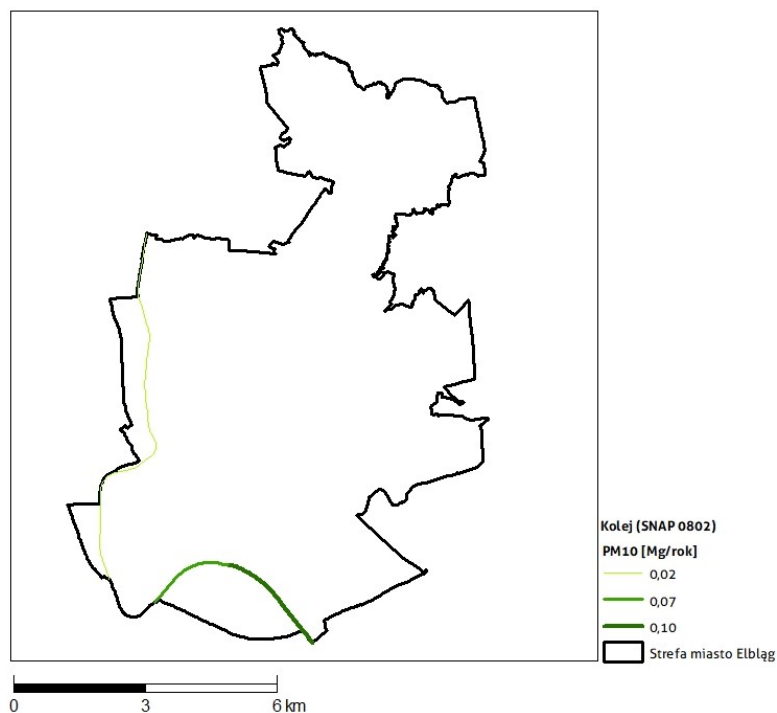
Rysunek 1-32 Rozmieszczenie oraz ładunki emisji pyłu zawieszonego PM10 w transporcie kolejowym (SNAP 0802) w strefie miasto Elbląg w 2018 r.
