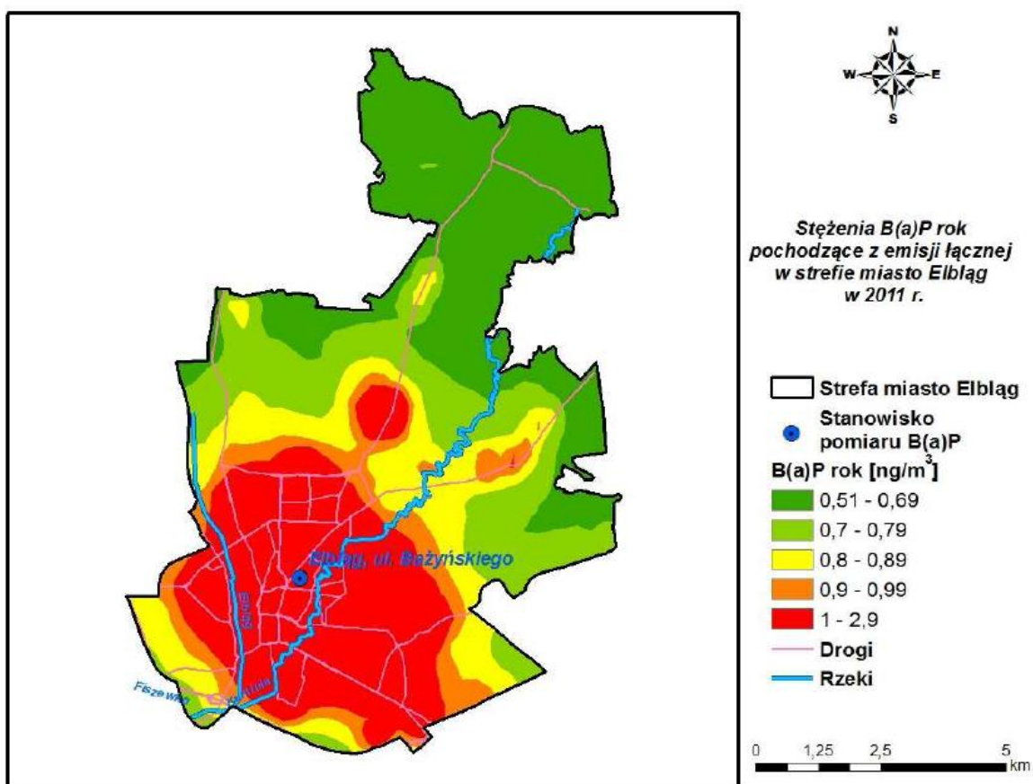
Rysunek 5-4 Stężenia B(a)P o okresie uśredniania wyników w skali roku w mieście Elblągu pochodzące z łącznej emisji wszystkich typów w 2011 roku
