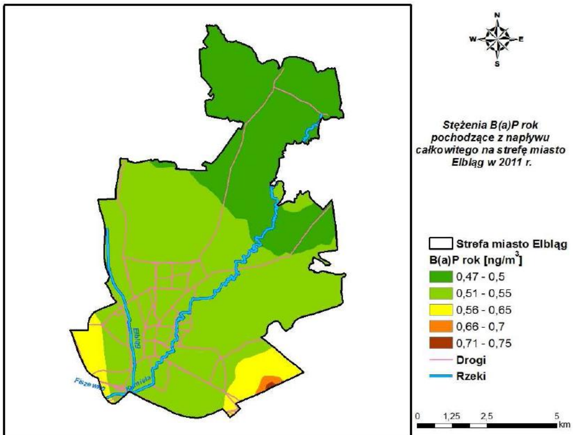
Rysunek 5-1 Stężenia B(a)P o okresie uśredniania wyników w skali roku w mieście Elblągu pochodzące z emisji punktowej w 2011 roku
